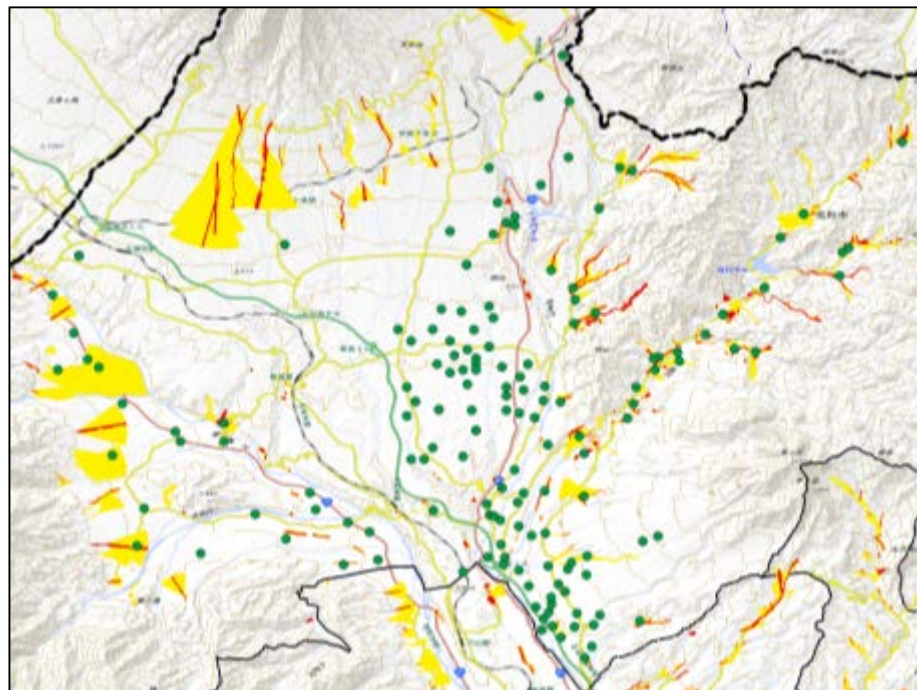
集落情報に土砂災害警戒区域を重ねる
