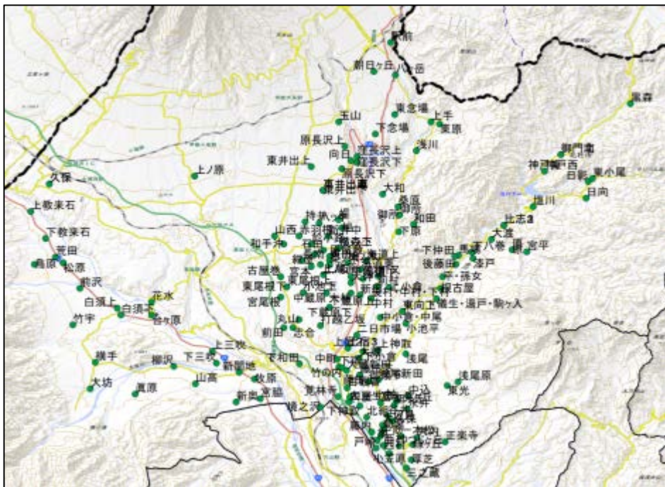
集落位置情報
